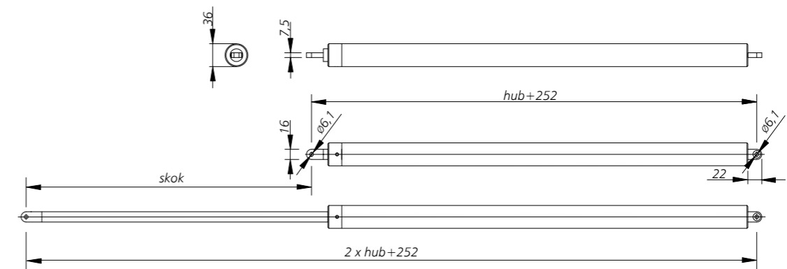
Abb. 105 - Abmessungen des elektrischen Spindeltriebs Typ S [mm]
