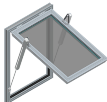
Abb. 90 - mcr OSO THERM 75 RWA-Fenster mit zwei Spindelantrieben Typ G mit versetzter Aufhängung
