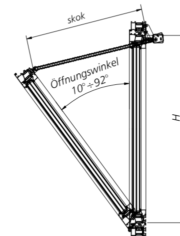
Abb. 34 - Vertikalschnitt A-A durch ein RWA-Fenster mcr OSO THERM 75 in geöffneter Position
