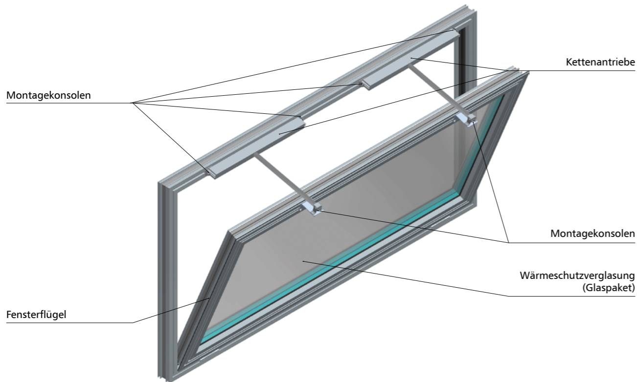
Abb. 64 - mcr OSO THERM 75 RWA-Fenster einwärts öffnend mit zwei Kettenantrieben
