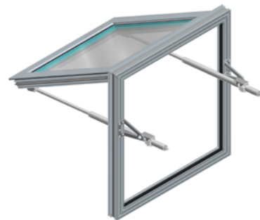
Abb. 42 - mcr OSO THERM 75 RWA-Fenster mit zwei Spindelantrieben Typ S mit versetzter Aufhängung
