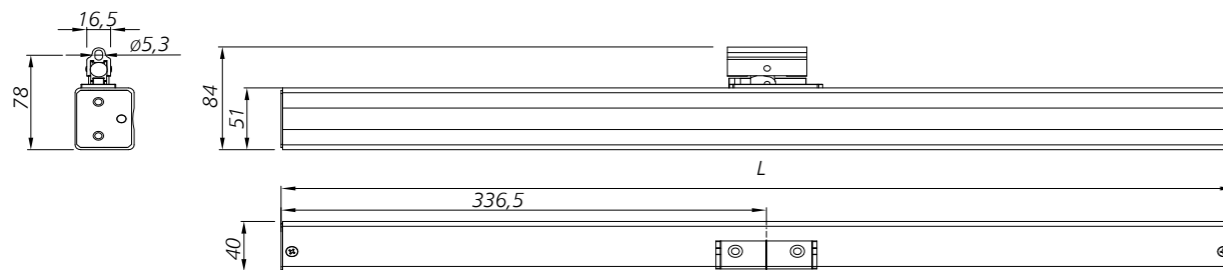
Abb. 115 - Abmessungen des Kettenträgers HCVA, Abmessungen [mm]
