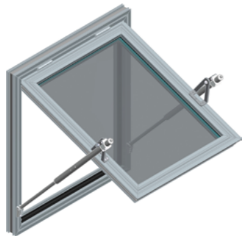
Abb. 89 - mcr OSO THERM 75 RWA-Fenster mit zwei Spindelantrieben Typ S mit versetzter Aufhängung
