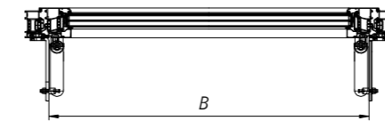
Abb. 20 - Horizontalschnitt B-B durch ein RWA-Fenster mcr OSO THERM 75 in geschlossener Position
