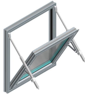
Abb. 85 - mcr OSO THERM 75 RWA-Fenster mit zwei Spindelantrieben Typ S mit versetzter Aufhängung
