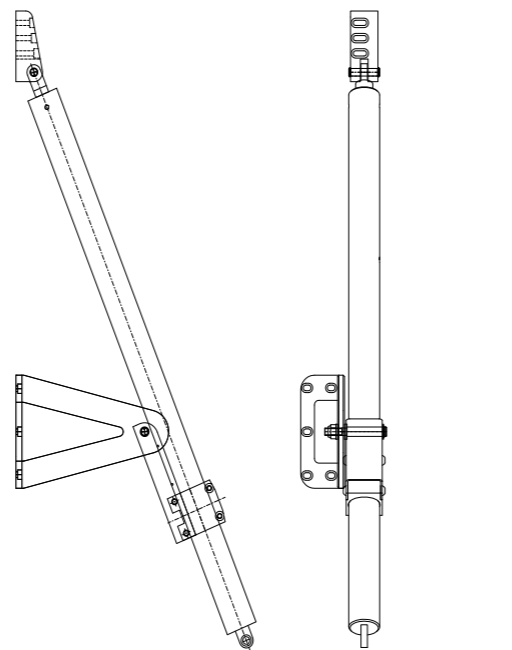
Abb. 111 - Spindelzylinder Typ S mit montierten oberen und unteren Konsolen mit versetztem Drehpunkt
