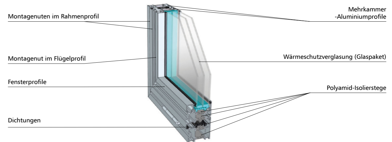
Abb. 48 - Schnitt durch ein einwärts öffnendes Rauchabzugsfenster
