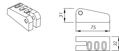
Abb. 106 - Obere Montagekonsole zur Montage des Spindeltriebs Typ S am RWA Fenster, Abmessungen [mm]
