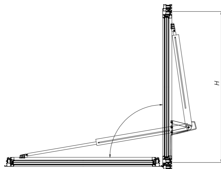
Abb. 25 - Vertikalschnitt A-A durch ein mcr OSO THERM 75 RWA-Fenster in geöffneter Position
