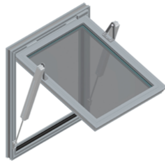
Abb. 56 - mcr OSO THERM 75 RWA-Fenster mit zwei Spindelantrieben Typ G
