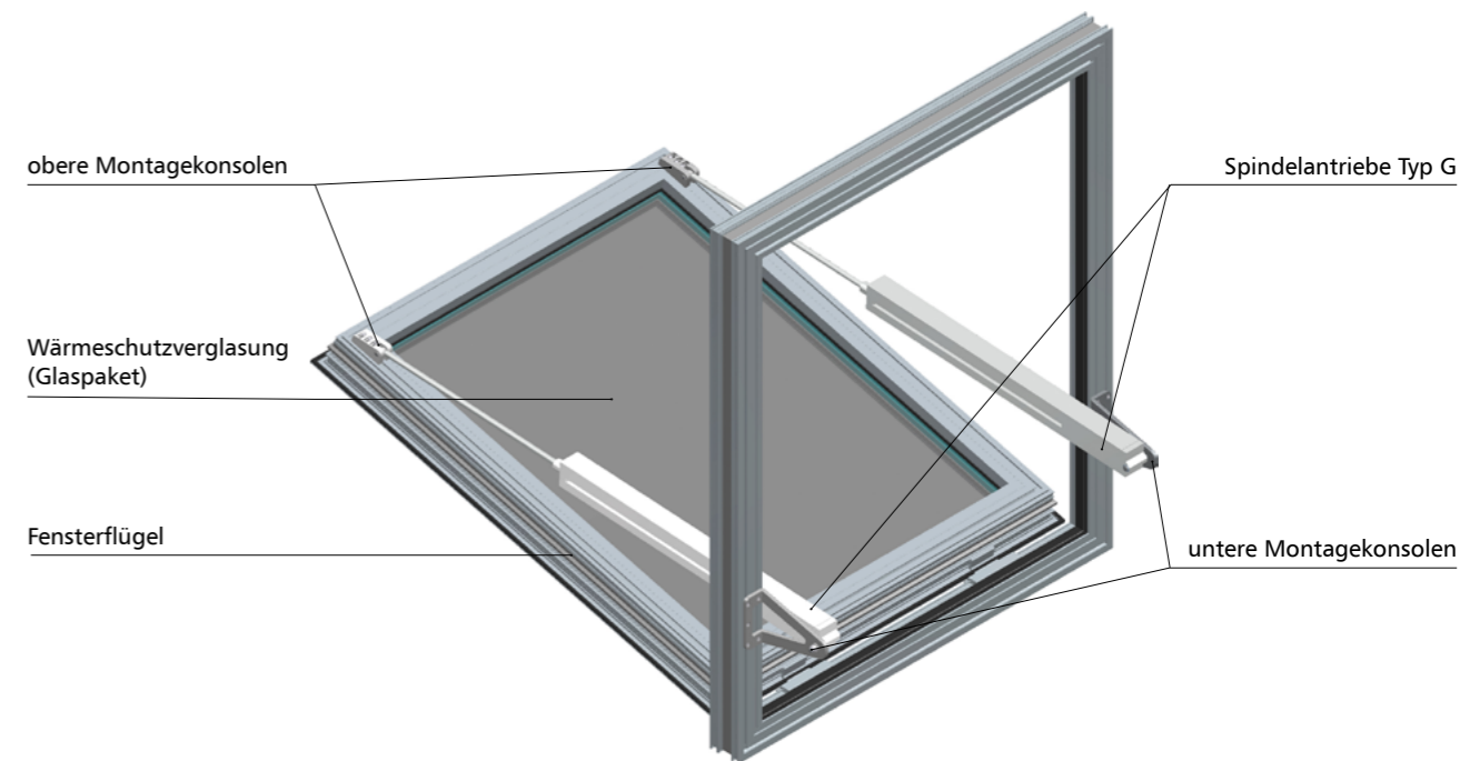
Abb. 14 - mcr OSO THERM 75 RWA-Fenster auswärts öffnend mit zwei Spindeltrieben Typ G
