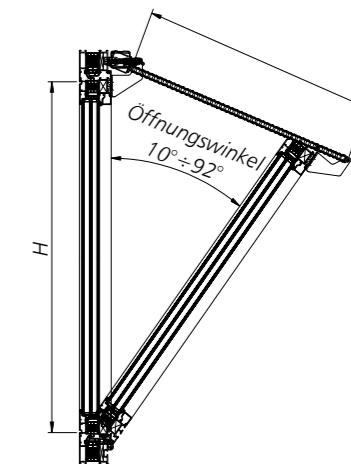
Abb. 81 - Horizontalschnitt B-B durch ein mcr OSO THERM 75 RWA-Fenster in geschlossener Position
