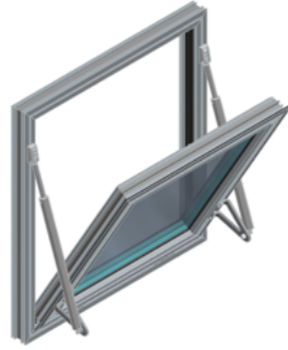
Abb. 83 - mcr OSO THERM 75 RWA-Fenster mit zwei Spindelantrieben Typ S
