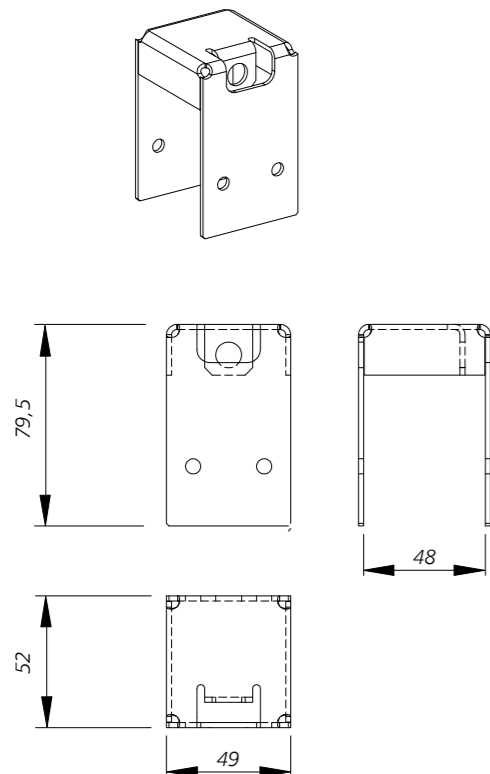
Abb. 103 - Montagekonsole zur stufenlosen Montage des Spindeltriebs Typ G mit regulierbaren (mittlerer) Aufhängung am RWA Fenster, Abmessungen [mm]
