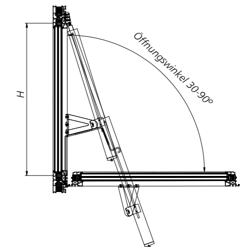
Abb. 69 - Horizontalschnitt B-B durch ein mcr OSO THERM 75 RWA-Fenster in geschlossener Position
