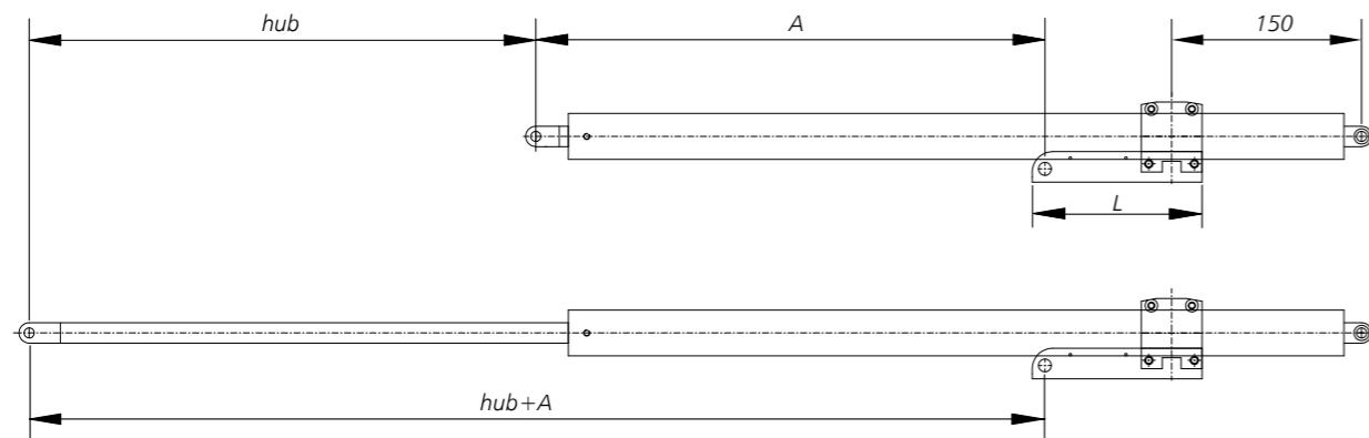
Abb. 109 - Abmessungen des elektrischen Spindeltriebs Typ S mit versetzter Aufhängung [mm]
