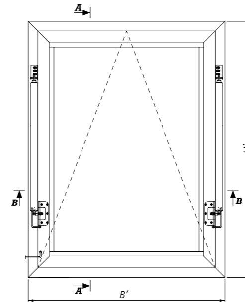
Abb. 65 - Innenansicht von einem mcr OSO THERM 75 RWA-Fenster mit Spindelantrieben Typ S in geschlossener Position
