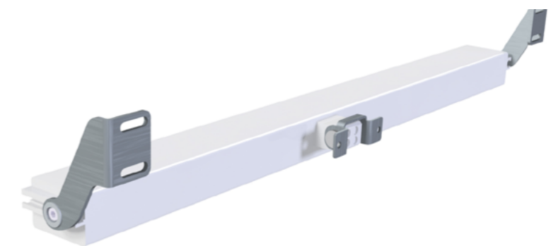
Abb. 113 - HCV-Kettenantrieb mit Konsolen für nach außen öffnendes Fenster
