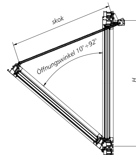
Abb. 31 - Vertikalschnitt A-A durch ein RWA-Fenster mcr OSO THERM 75 in geöffneter Position
