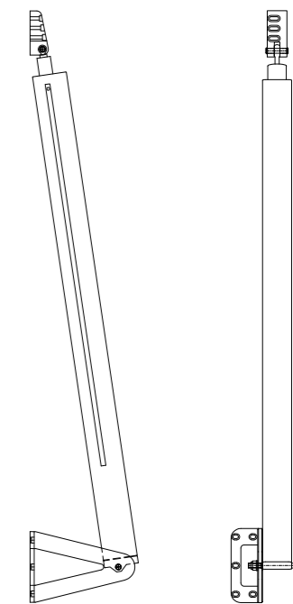
Abb. 101 - Spindeltrieb Typ G mit montierter oberer und unterer Montagekonsole
