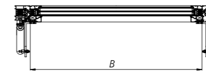
Abb. 67 - Horizontalschnitt B-B durch ein mcr OSO THERM 75 RWA-Fenster in geschlossener Position
