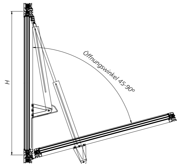
Abb. 72 - Vertikalschnitt A-A durch ein mcr OSO THERM 75 RWA-Fenster in geöffneter Position
