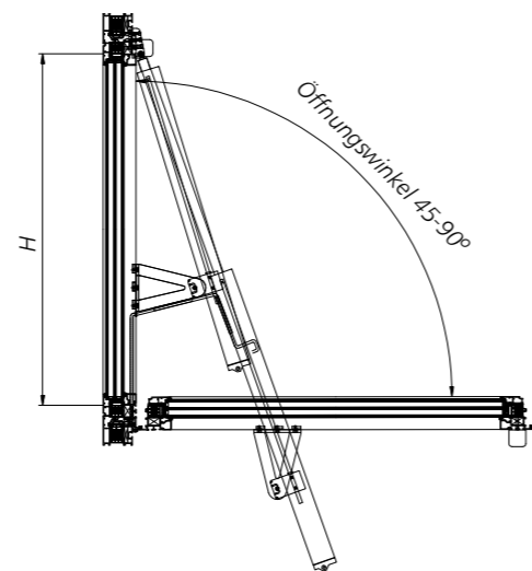
Abb. 75 - Vertikalschnitt A-A durch ein mcr OSO THERM 75 RWA-Fenster mit versetzter Aufhängung in geöffneter Position
