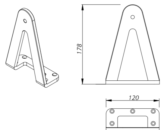
Abb. 100 - Untere Montagekonsole zur Montage des Spindeltriebs Typ G am RWA-Fenster, Abmessungen [mm]
