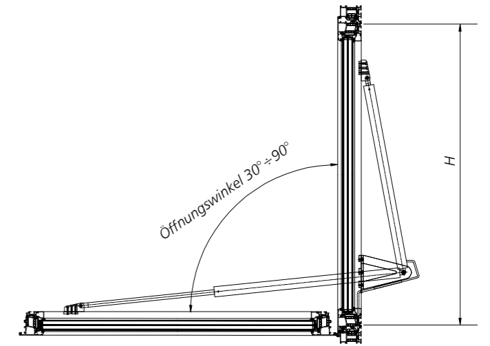
Abb. 19 - Vertikalschnitt A-A durch ein mcr OSO THERM 75 RWA-Fenster in geöffneter Position
