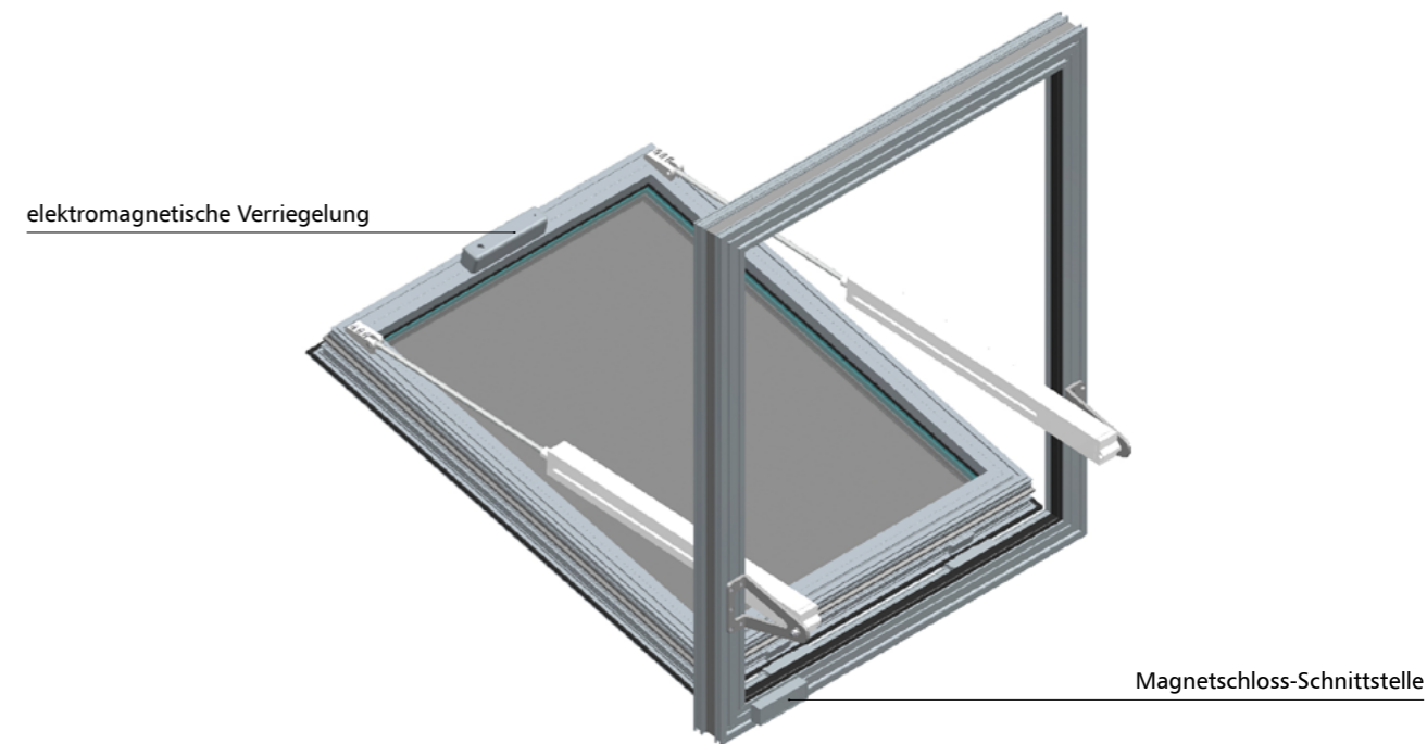
Abb. 15 - mcr OSO THERM 75 RWA-Fenster auswärts öffnend mit zwei Spindeltrieben Typ G, mit elektrischem Magnetschloss und Schnittstelle
