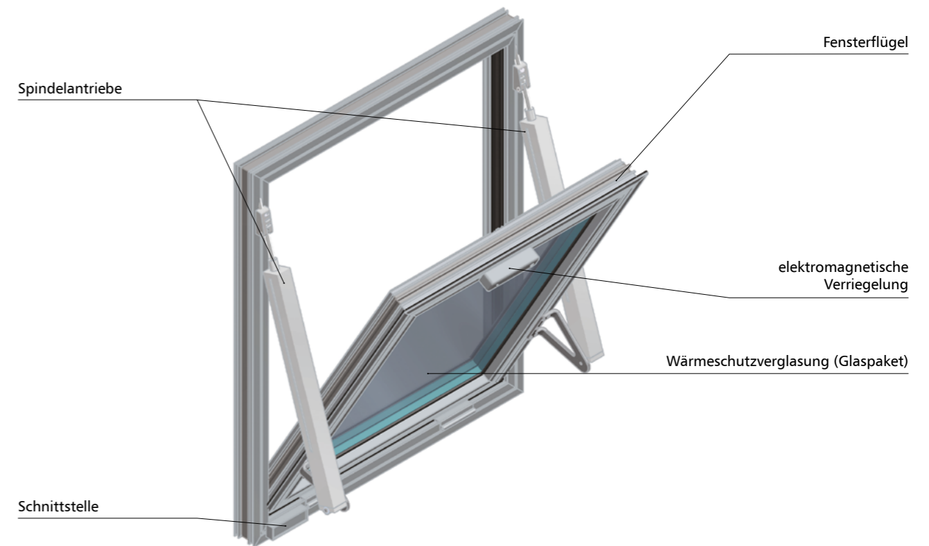
Abb. 62 - mcr OSO THERM 75 RWA-Fenster einwärts öffnend mit zwei Spindelantrieben mit elektrischem Magnetschloss und Schnittstelle
