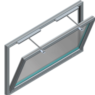
Abb. 54 - mcr OSO THERM 75 RWA-Fenster mit zwei Kettenantrieben Typ HCV mit versetzter Aufhängung
