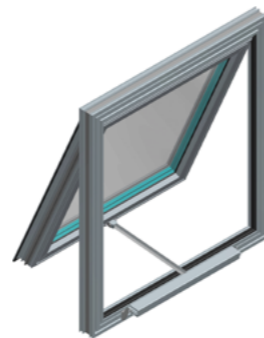
Abb. 10 - mcr OSO THERM 75 RWA-Fenster mit einem Kettenantrieb Typ HCV
