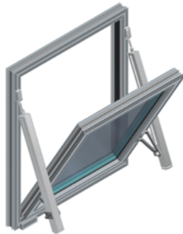
Abb. 53 - mcr OSO THERM 75 RWA-Fenster mit zwei Spindelantrieben Typ G mit versetzter Aufhängung
