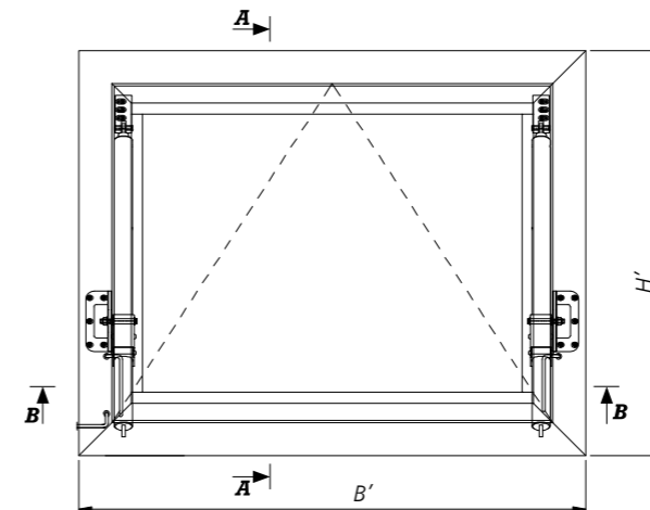
Abb. 21 - Innenansicht von einem mcr OSO THERM 75 RWA-Fenster mit Spindelantrieben Typ S mit versetzter Aufhängung in geschlossener Position
