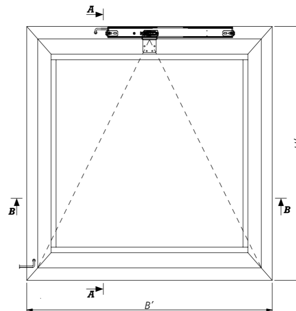
Abb. 77 - Innenansicht von einem mcr OSO THERM 75 RWA-Fensters mit dem HCV-Kettenantrieb in geschlossener Position
