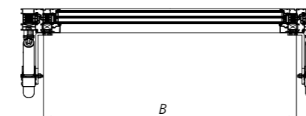
Abb. 70 - Vertikalschnitt A-A durch ein mcr OSO THERM 75 RWA-Fenster mit versetzter Aufhängung in geöffneter Position
