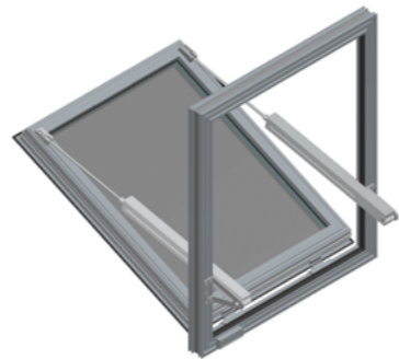
Abb. 3 - mcr OSO THERM 75 RWA-Fenster mit zwei Spindeltrieben Typ G
