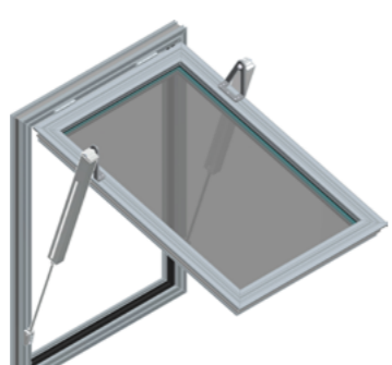
Abb. 59 - mcr OSO THERM 75 RWA-Fenster mit zwei Spindelantrieben Typ G mit versetzter Aufhängung
