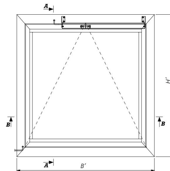
Abb. 30 - Innenansicht von einem mcr OSO THERM 75 RWA-Fenster mit dem HCV-Kettenantrieb in geschlossener Position
