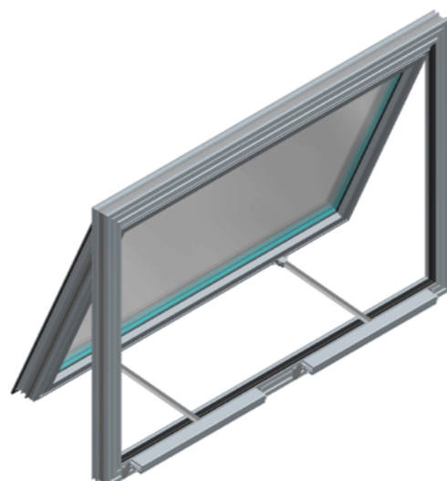
Abb. 47 - mcr OSO THERM 75 RWA-Fenster mit zwei Kettenantrieben HCV
