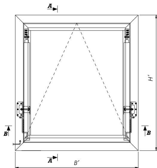
Abb. 27 - Innenansicht mcr OSO THERM 75 RWA-Fenster mit Spindeltrieben Typ G mit versetzter Aufhängung in geschlossener Position
