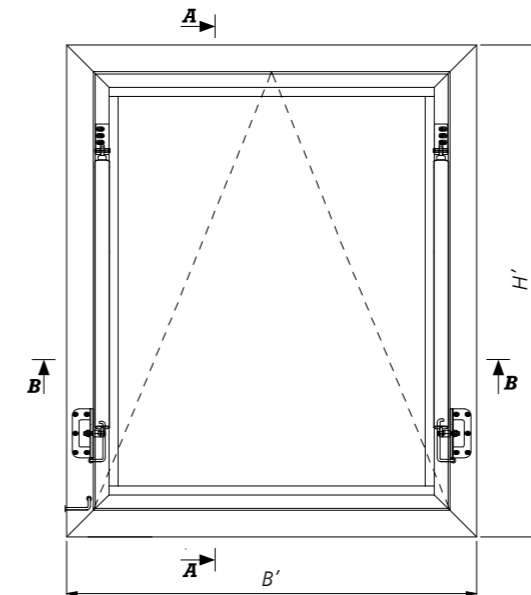
Abb. 18 - Innenansicht von einem mcr OSO THERM 75 RWA-Fenster mit Spindelantrieben Typ S in geschlossener Position
