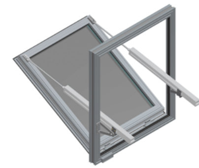
Abb. 6 - mcr OSO THERM 75 RWA-Fenster mit zwei Spindeltrieben Typ G mit versetzter Aufhängung
