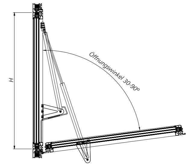
Abb. 66 - Vertikalschnitt A-A durch ein mcr OSO THERM 75 RWA-Fenster in geöffneter Position
