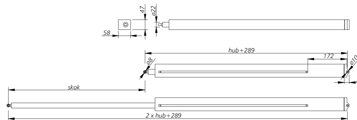
Abb. 98 - Abmessungen des elektrischen Spindeltriebs Typ G [mm]
