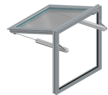
Abb. 9 - mcr OSO THERM 75 RWA-Fenster mit zwei Spindeltrieben Typ G
