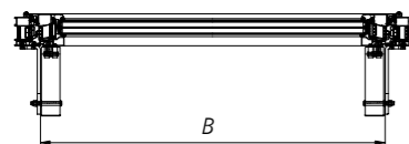
Abb. 26 - Horizontalschnitt B-B durch ein RWA-Fenster mcr OSO THERM 75 in geschlossener Position
