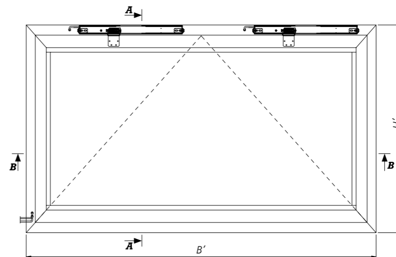
Abb. 80 - Innenansicht von einem mcr OSO THERM 75 RWA-Fensters mit zwei HCV-Kettenantrieben in geschlossener Position
