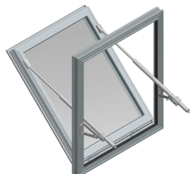
Abb. 5 - mcr OSO THERM 75 RWA-Fenster mit zwei Spindeltrieben Typ S mit versetzter Aufhängung
