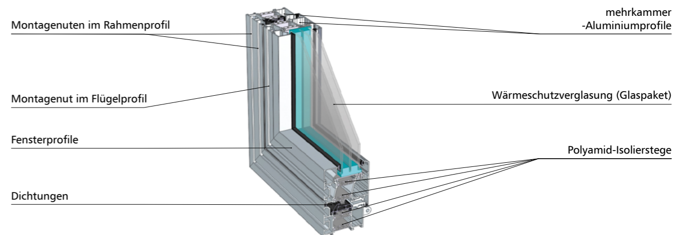
Abb. 1 - Schnitt durch ein auswärts öffnendes Rauchabzugsfenster
