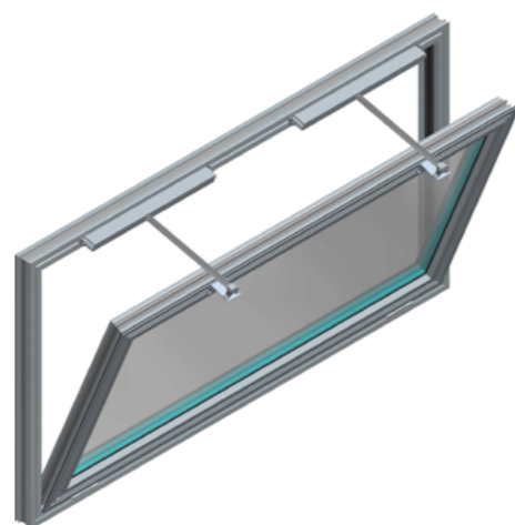
Abb. 92 - mcr OSO THERM 75 RWA-Fenster mit zwei Kettenantriebe HCV
