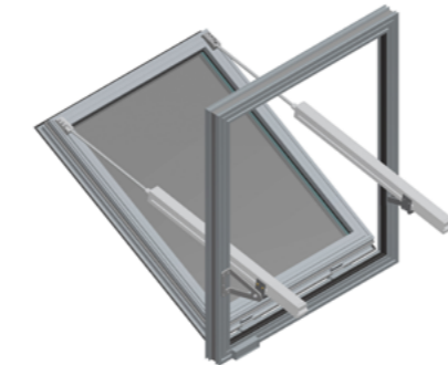
Abb. 39 - mcr OSO THERM 75 RWA-Fenster mit zwei Spindelantrieben Typ G mit versetzter Aufhängung
