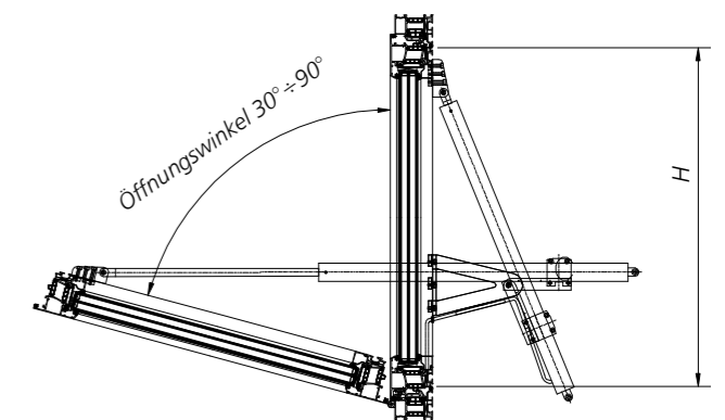
Abb. 22 - Horizontalschnitt B-B durch ein mcr OSO THERM 75 RWA-Fenster in geschlossener Position
