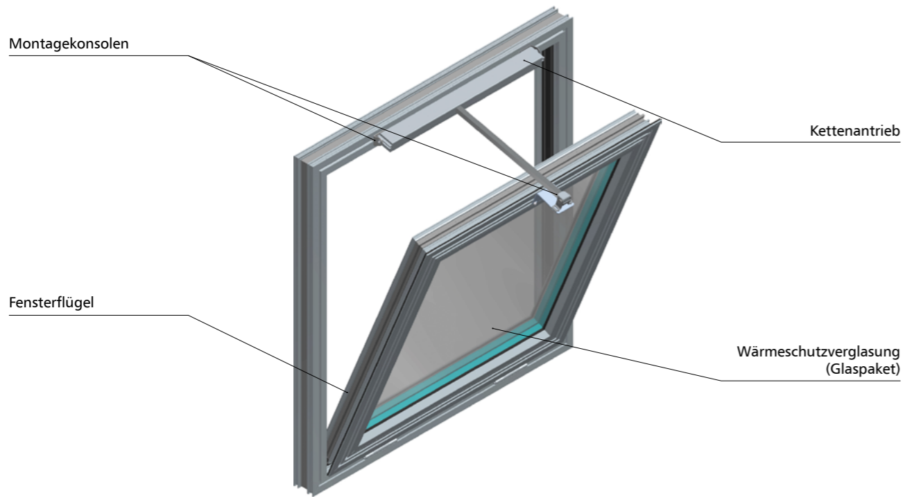
Abb. 63 - mcr OSO THERM 75 RWA-Fenster einwärts öffnend mit einem Kettenantrieb
