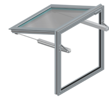
Abb. 41 - mcr OSO THERM 75 RWA-Fenster mit zwei Spindelantrieben Typ G
