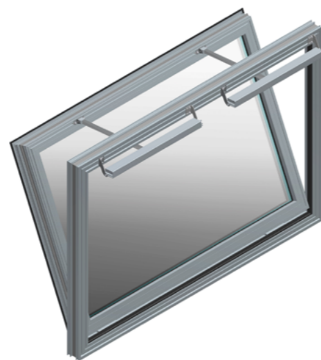
Abb. 45 - mcr OSO THERM 75 RWA-Fenster mit zwei Kettenantrieben HCV
