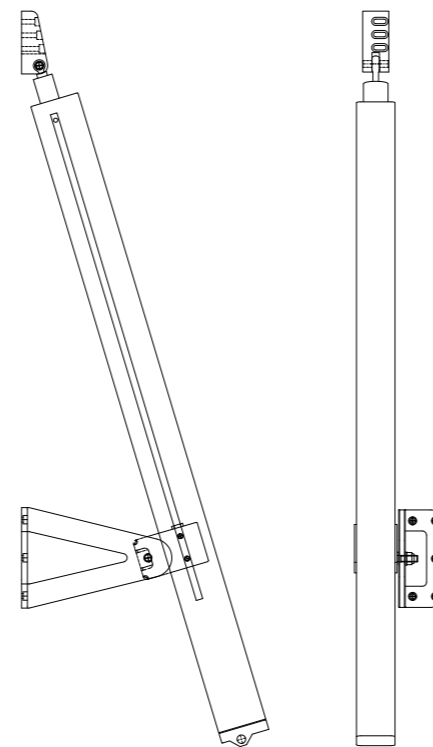
Abb. 104 - Spindeltrieb Typ G mit montierter oberer und unterer Montagekonsole mit versetzter (mittlerer) Aufhängung
