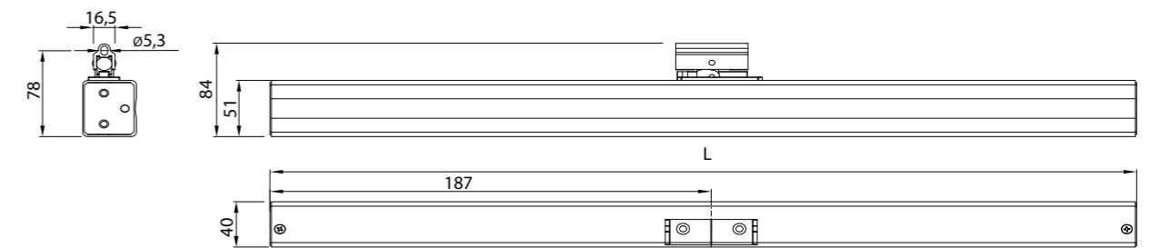
Abb. 112 - Abmessungen des Elektrokettenantriebs HCV, Abmessungen [mm]
