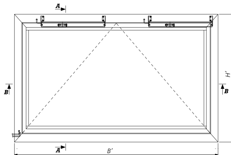
Abb. 33 - Innenansicht von einem mcr OSO THERM 75 RWA-Fenster mit zwei HCV-Kettenantrieben in geschlossener Position
