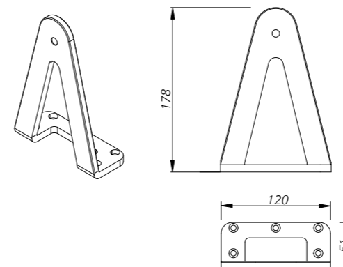
Abb. 106 - Obere Montagekonsole zur Montage des Spindeltriebs Typ S am RWA Fenster, Abmessungen [mm]
