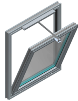
Abb. 51 - mcr OSO THERM 75 RWA-Fenster mit Kettenantrieb Typ HCV
