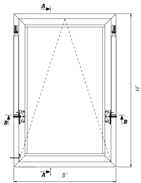
Abb. 71 - Innenansicht von einem mcr OSO THERM 75 RWA-Fenster mit Spindeltrieben Typ G in geschlossener Position
