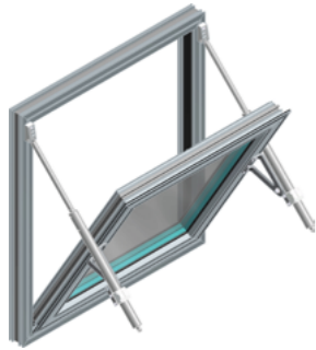
Abb. 52 - mcr OSO THERM 75 RWA-Fenster mit zwei Spindelantrieben Typ S mit versetzter Aufhängung
