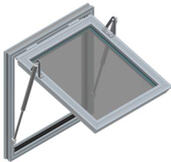
Abb. 87 - mcr OSO THERM 75 RWA-Fenster mit zwei Spindelantrieben Typ S
