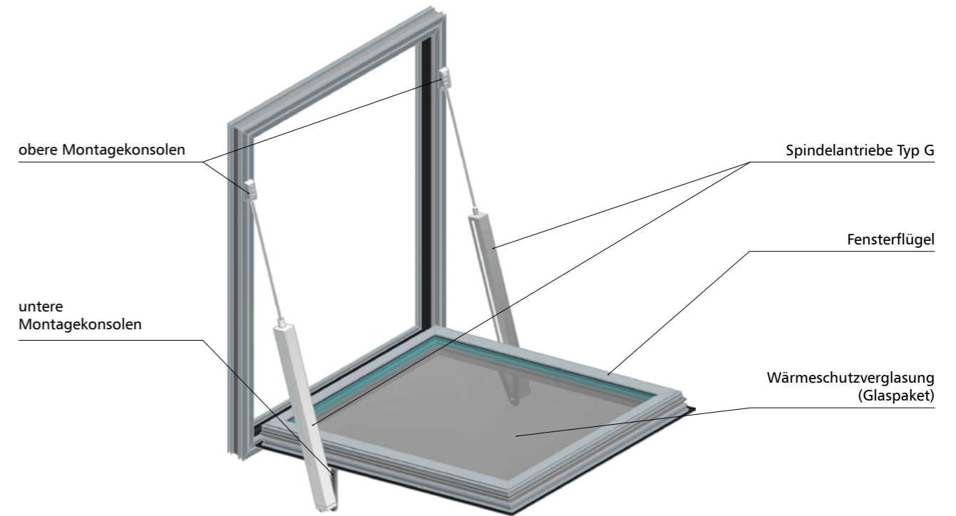
Abb. 61 - mcr OSO THERM 75 RWA-Fenster einwärts öffnend mit zwei Spindelantrieben
