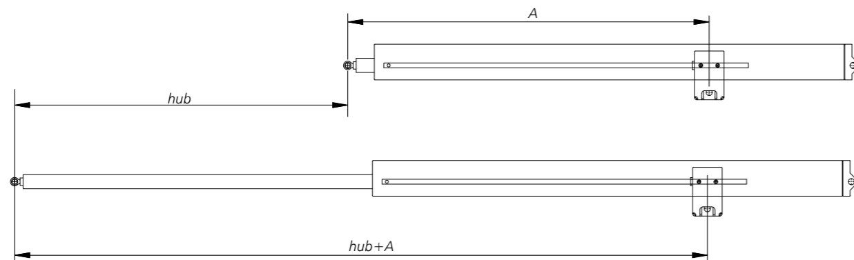
Abb. 102 - Abmessungen des Spindeltriebs Typ G mit versetzter (mittlerer) Aufhängung
