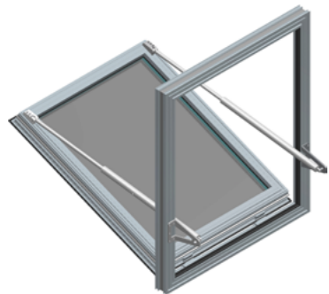
Abb. 2 - mcr OSO THERM 75 RWA-Fenster mit zwei Spindeltrieben Typ S
