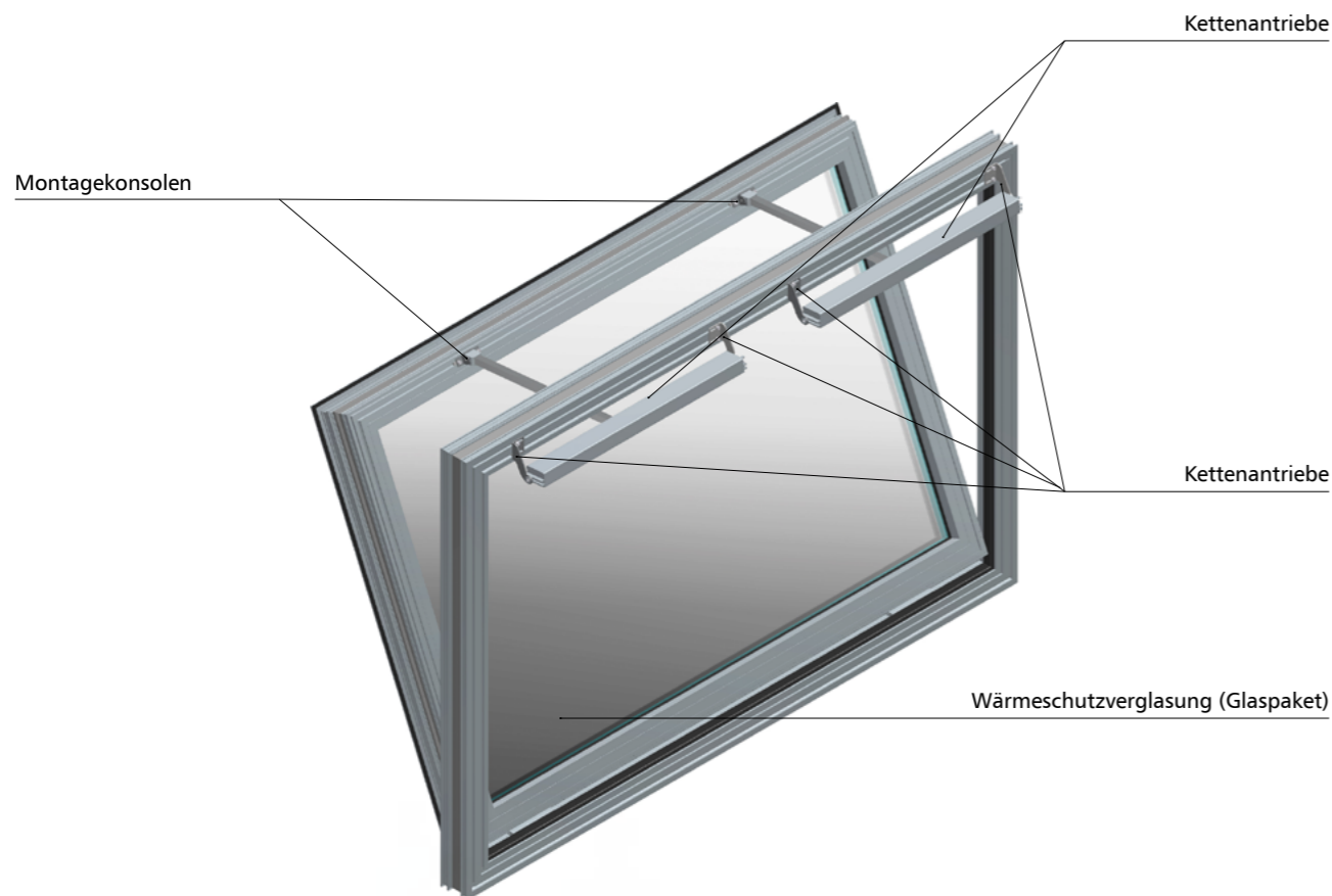
Abb. 17 - mcr OSO THERM 75 RWA-Fenster auswärts öffnend mit zwei Kettenantrieben
