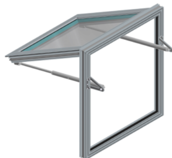
Abb. 8 - mcr OSO THERM 75 RWA-Fenster mit zwei Spindeltrieben Typ S
