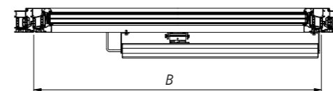
Abb. 32 - Horizontalschnitt B-B durch ein RWA-Fenster mcr OSO THERM 75 in geschlossener Position
