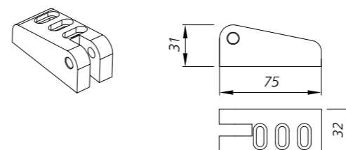
Abb. 99 - Obere Montagekonsole zur Montage des Spindeltriebs Typ G am RWA-Fenster, Abmessungen [mm]
