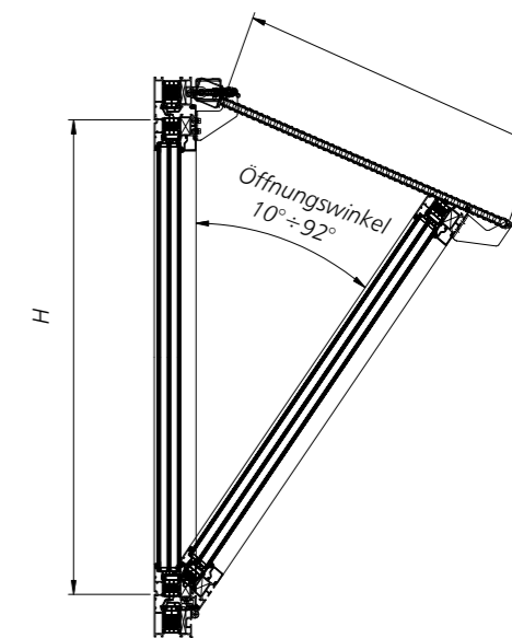
Abb. 78 - Vertikalschnitt A-A durch ein mcr OSO THERM 75 RWA-Fenster in geöffneter Position
