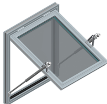
Abb. 58 - mcr OSO THERM 75 RWA-Fenster mit zwei Spindelantrieben Typ S mit versetzter Aufhängung
