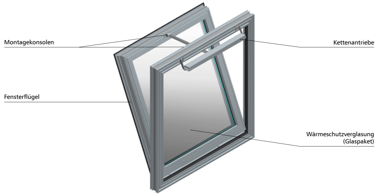
Abb. 16 - mcr OSO THERM 75 RWA-Fenster auswärts öffnend mit einem Kettenantrieb
