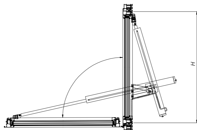
Abb. 28 - Vertikalschnitt A-A durch das mcr OSO THERM 75 RWA-Fenster mit versetzter Aufhängung in geöffneter Position
