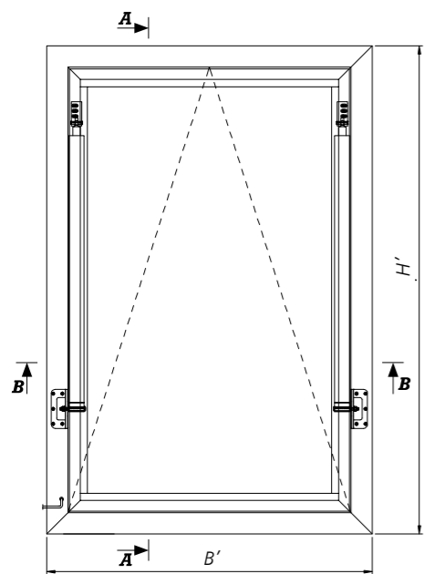
Abb. 24 - Innenansicht von einem mcr OSO THERM 75 RWA-Fenster mit Spindeltrieben Typ G in geschlossener Position
