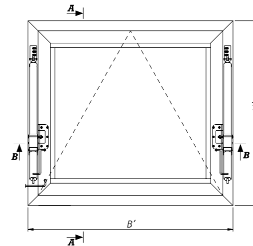
Abb. 68 - Innenansicht von einem mcr OSO THERM 75 RWA-Fenster mit Spindelantrieben Typ S mit versetzter Aufhängung in geschlossener Position
