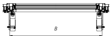
Abb. 29 - Horizontalschnitt B-B durch ein mcr OSO THERM 75 RWA-Fenster mit versetzter Aufhängung in geschlossener Position
