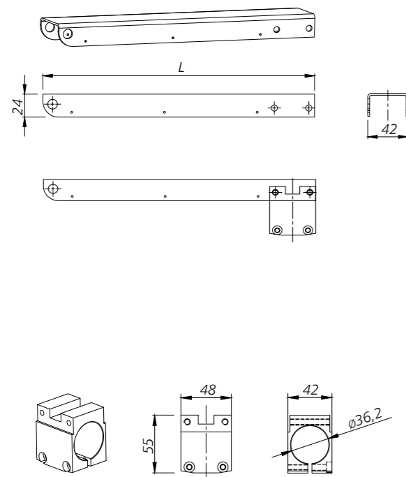
Abb. 110 - Klemmstück zur Montage des S-Spindeltriebs mit versetztem Drehpunkt am RWA-Fenster, Abmessungen [mm]
